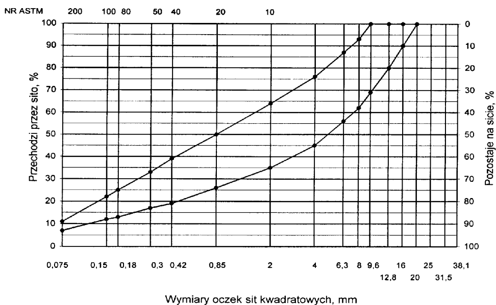
Rys. 2. Krzywe graniczne uziarnienia mieszanki mineralnej BA od 0 do 16mm, od 0 do 12,8 mm do warstwy ścieralnej nawierzchni drogi o obciążeniu ruchem KR I
